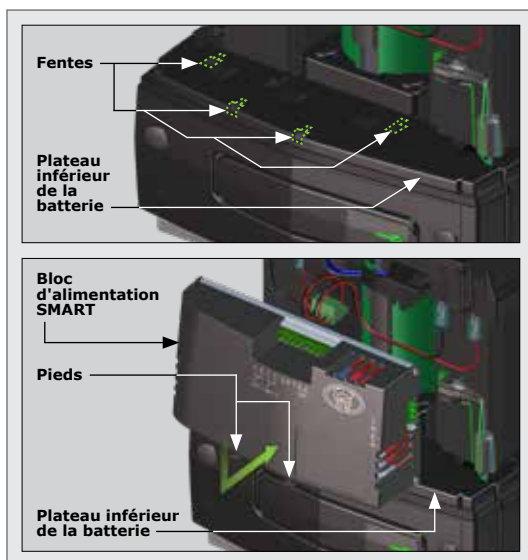
FIGURE 8. MISE EN PLACE DU BLOC D'ALIMENTATION SMART
