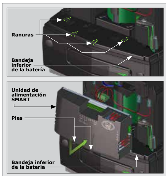
FIGURA 8. MONTAJE DE LA UNIDAD DE ALIMENTACIÓN SMART
