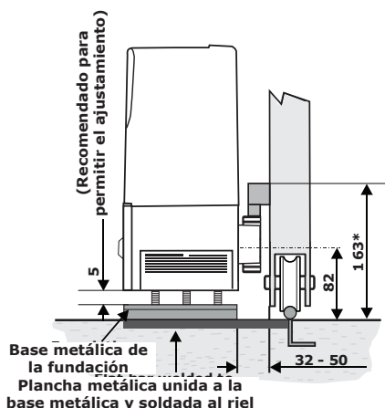
FIGURA 9A CREMALLERA DE RAZ, SOBRE EL PIÑÓN
