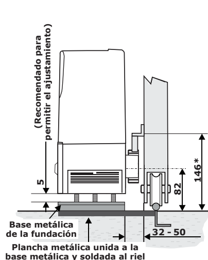
FIGURA 8A CREMALLERA DE ACERO EN CONTACTO SOBRE EL PIÑÓN
