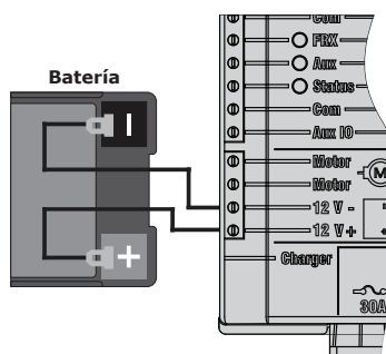
FIGURA 45 CONECCIÓN ESQUEMÁTICA DE LA BATERÍA
