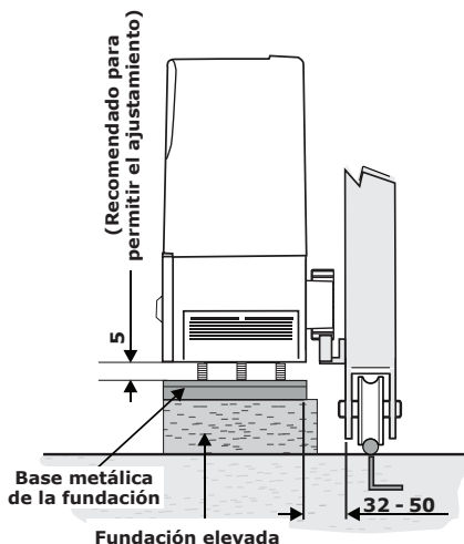
FIGURA 8B CREMALLERA DE ACERO EN CONTACTO POR DEBAJO DEL PIÑÓN
