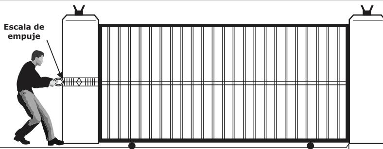
FIGURA 5 FUERZA DE PARTIDA Y FUERZA DE RECORRIDO
