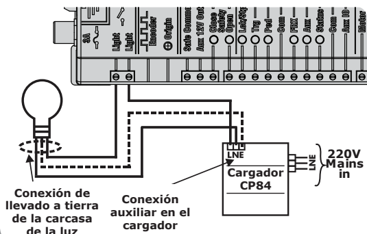
FIGURA 46 CONECCIÓN ESQUEMÁTICA DE LA LUZ
