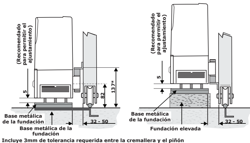
FIGURA 10A CREMALLERA DE NYLON CON SOPORTE DE ACERO ANGULADO, SOBRE EL PIÑÓN
