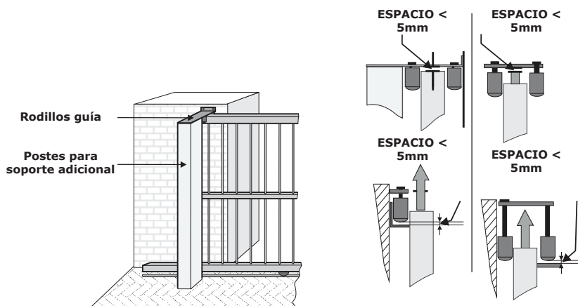
FIGURA 4 MONTANDO LOS RODILLOS GUÍAS
