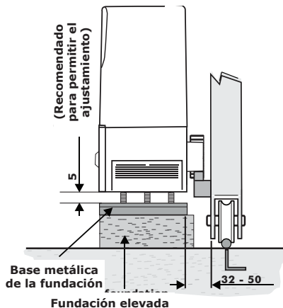
FIGURA 9B CREMALLERA DE RAZ, POR DEBAJO DEL PIÑÓN
