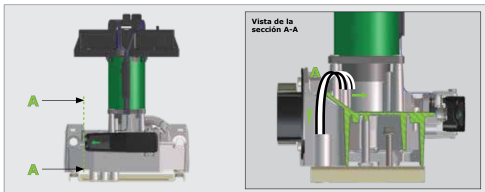
FIGURA 37. ENRUTAMIENTO DE CABLES PARA NUEVAS INSTALACIONES
