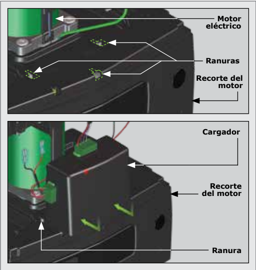
FIGURA 54. INSTALACIÓN DEL CARGADOR
