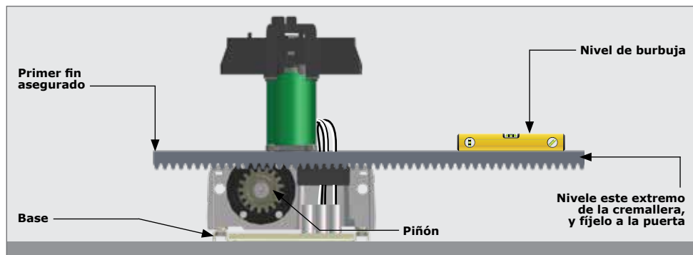
FIGURA 47. CREMALLERA Y MOTOR DESDE LA PERSPECTIVA DE LA PUERTA
