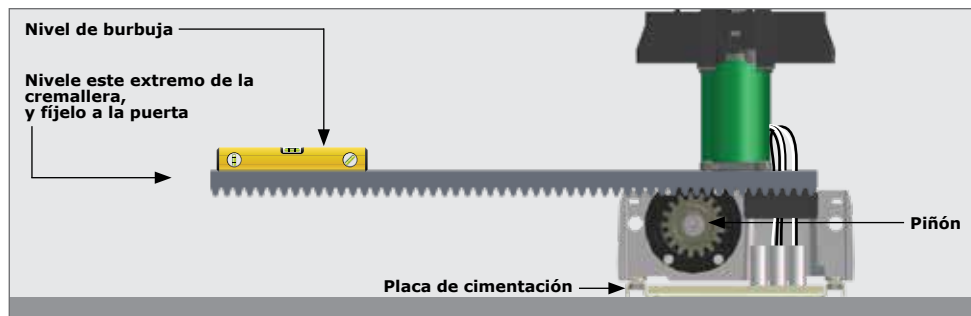
FIGURA 46. CREMALLERA Y MOTOR DESDE LA PERSPECTIVA DE LA PUERTA
