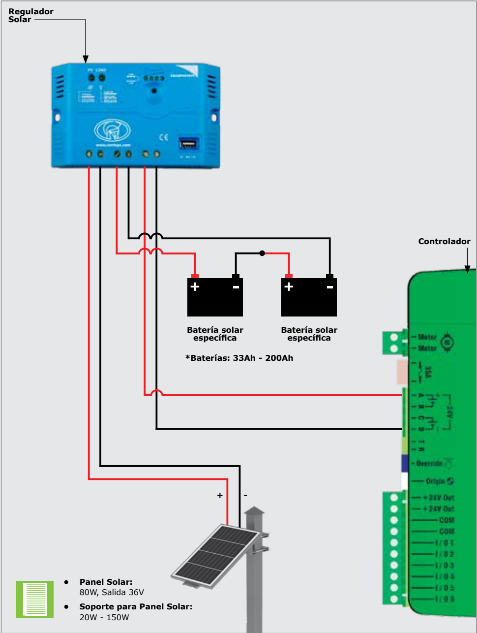
FIGURA 79. UN PANEL SOLAR INDIVIDUAL
