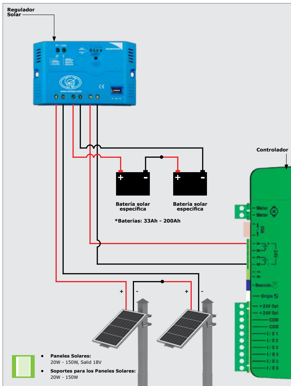
FIGURA 80. DOS PANELES SOLARES
