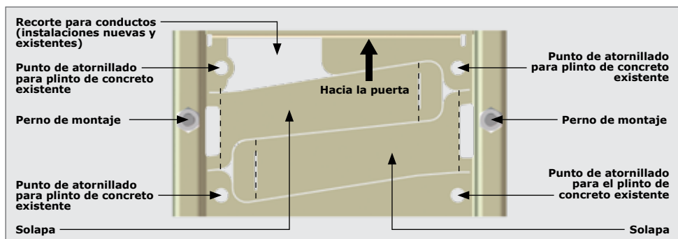
FIGURA 18. MONTAJE DE LA PLACA DE CIMENTACIÓN - VISTA SUPERIOR
