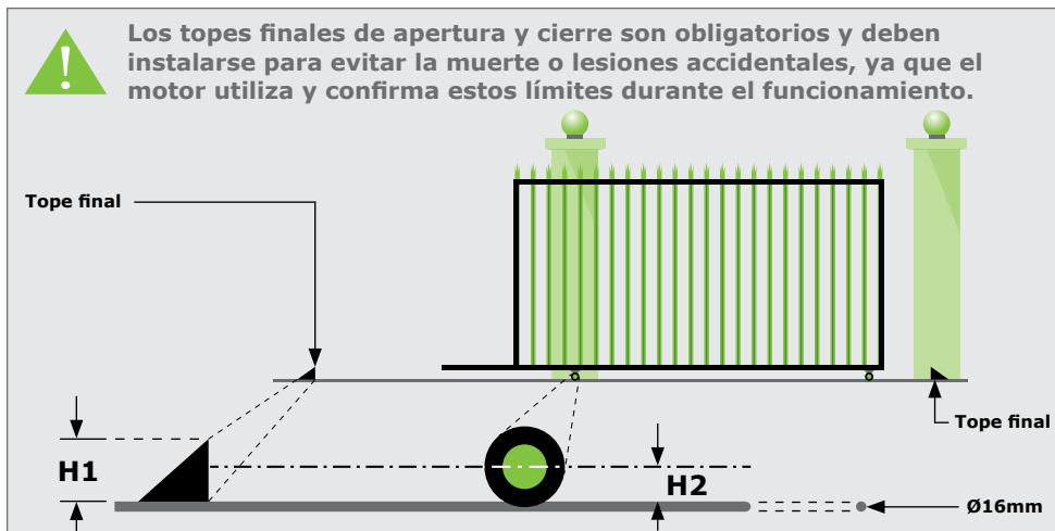
FIGURA 4. TOPES FINALES
