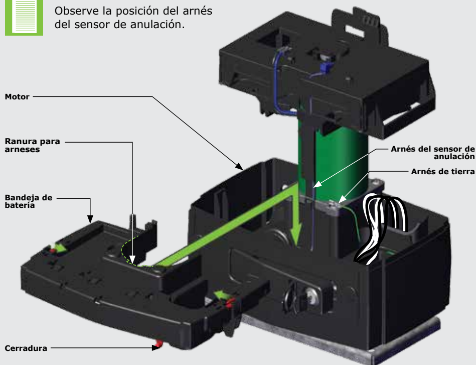
FIGURA 71. PONER LA BANDEJA INFERIOR DE LA BATERÍA
