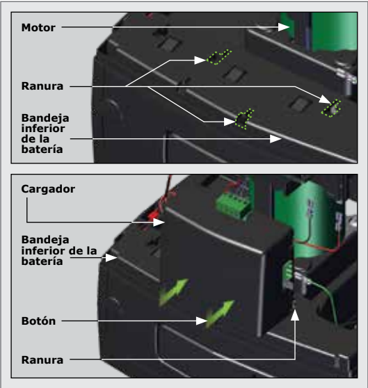
FIGURA 72. REMPLAZO DE LA BATERÍA
