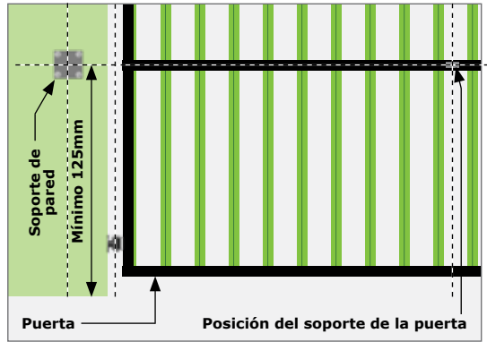
FIGURA 29. ALTURA DEL SOPORTE DE PARED
