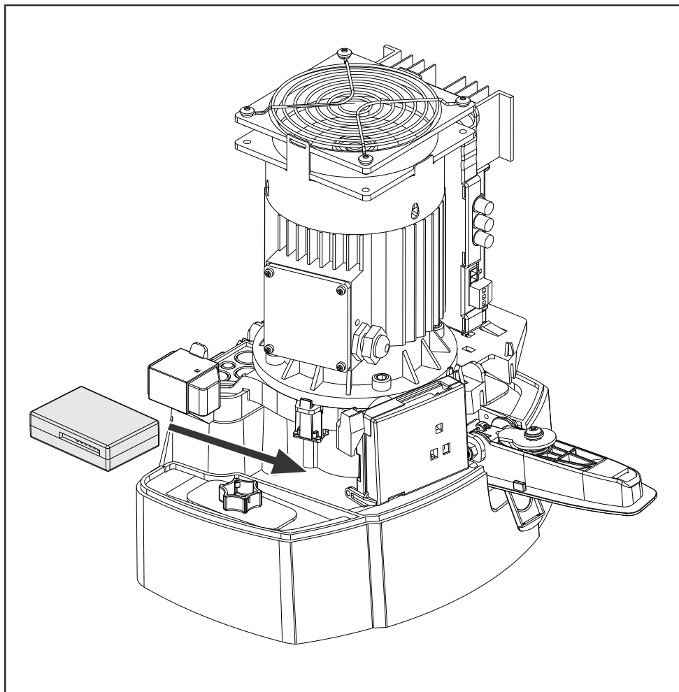
Figure 24 Installation du récepteur
