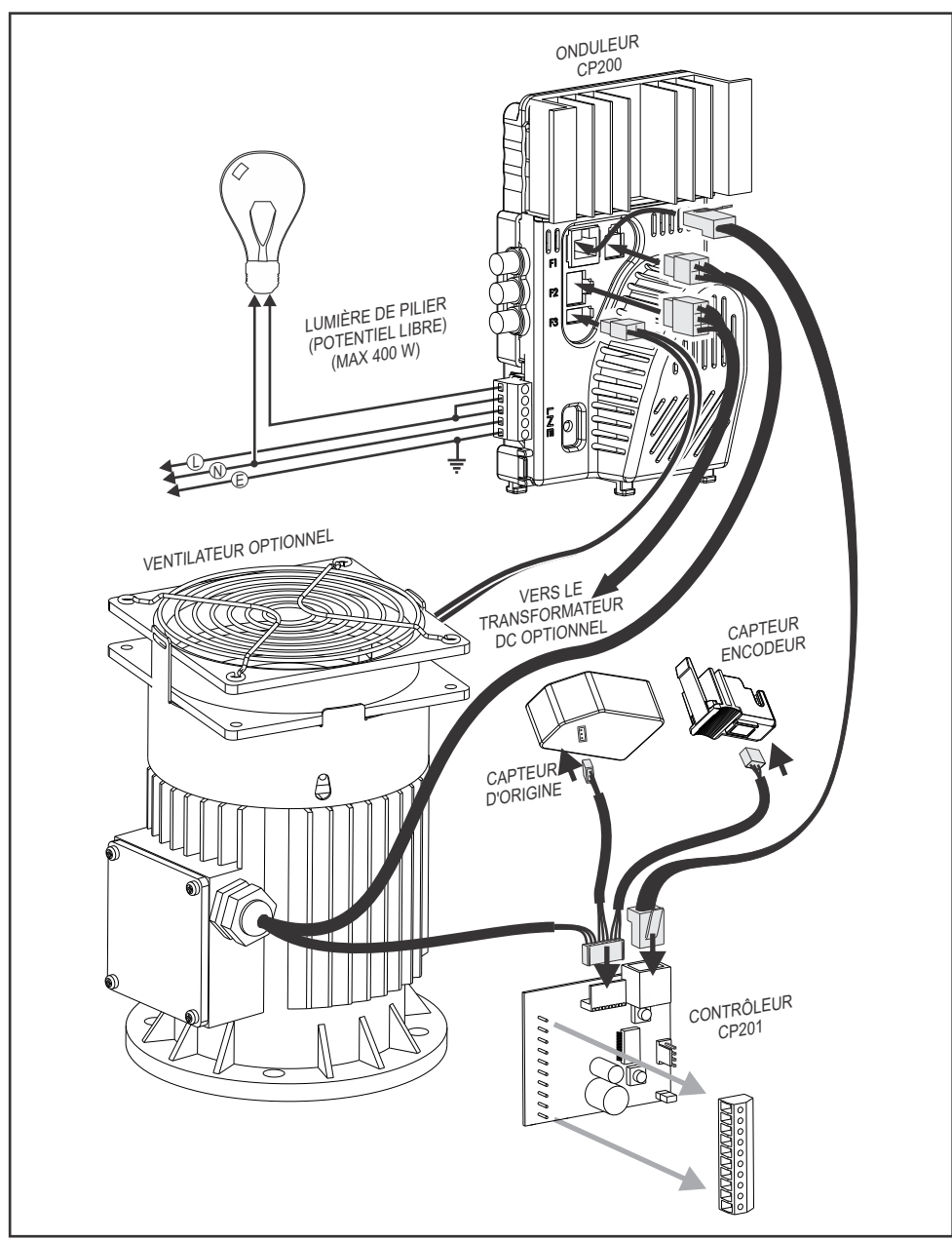
Figure 27 Interconnections des câbles de l'A10
