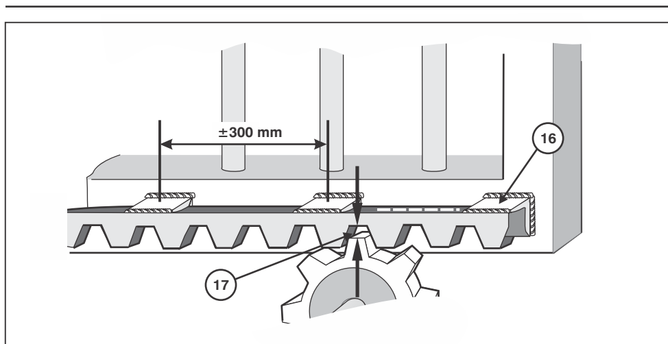
Figure 18 Montage de la crémaillère
