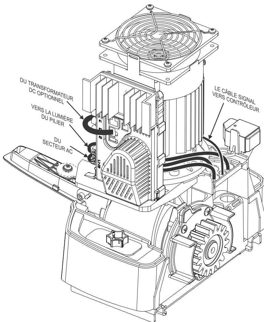
Figure 26 Routage des câbles de l'A10
