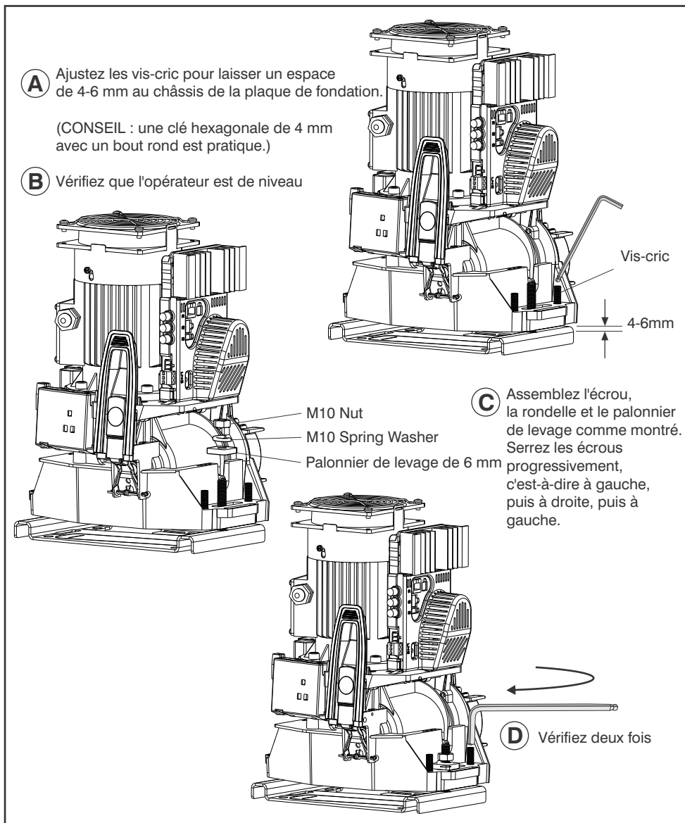
Figure 16 Détails du montage de la boîte de vitesses
