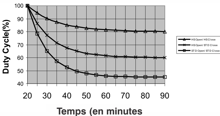
Figure 2 Courbes de rapport de cycle
